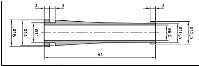
Anti kink grommet (15-633)
